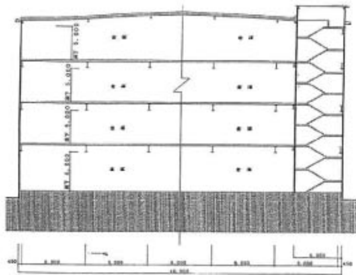
A-A' 断面图 1/300
