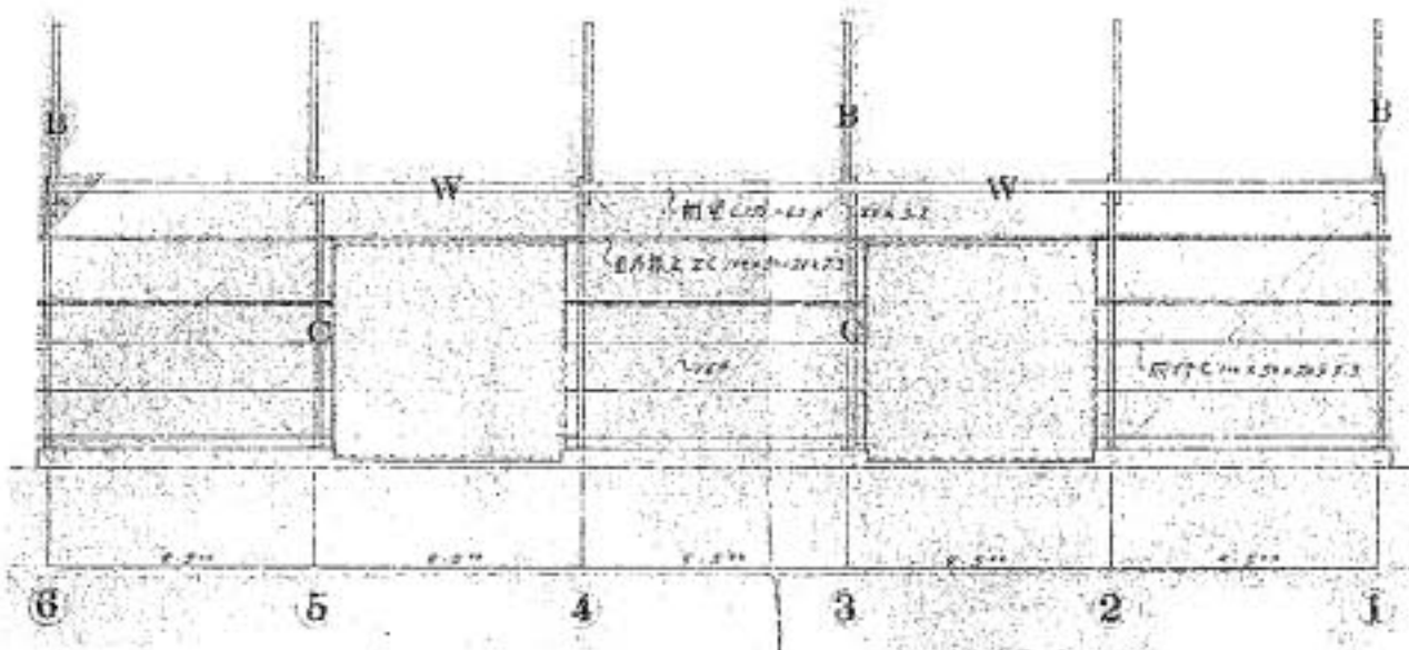
A 通轴 剖面图 1/100
