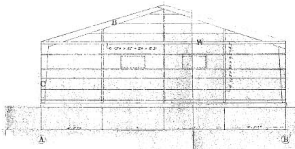
I 通轴 剖面图 1/100
