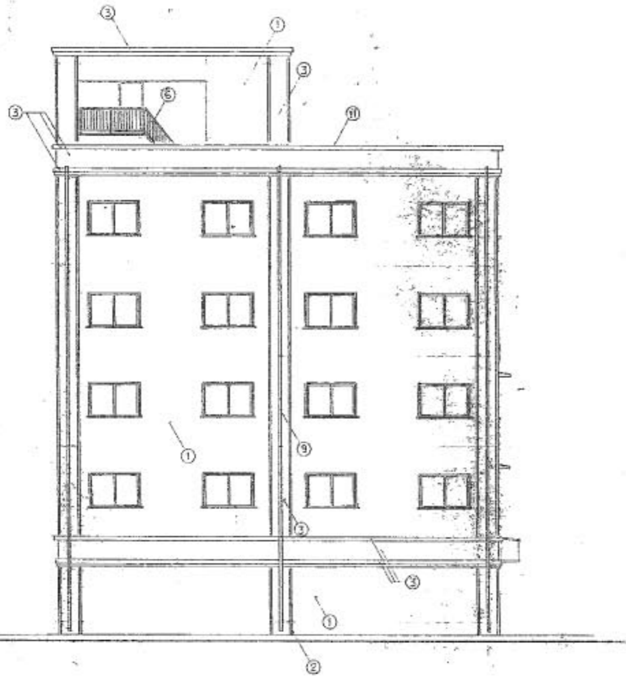
南立面图 1/100
