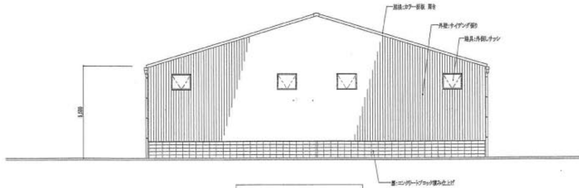
南立面図 1:100
